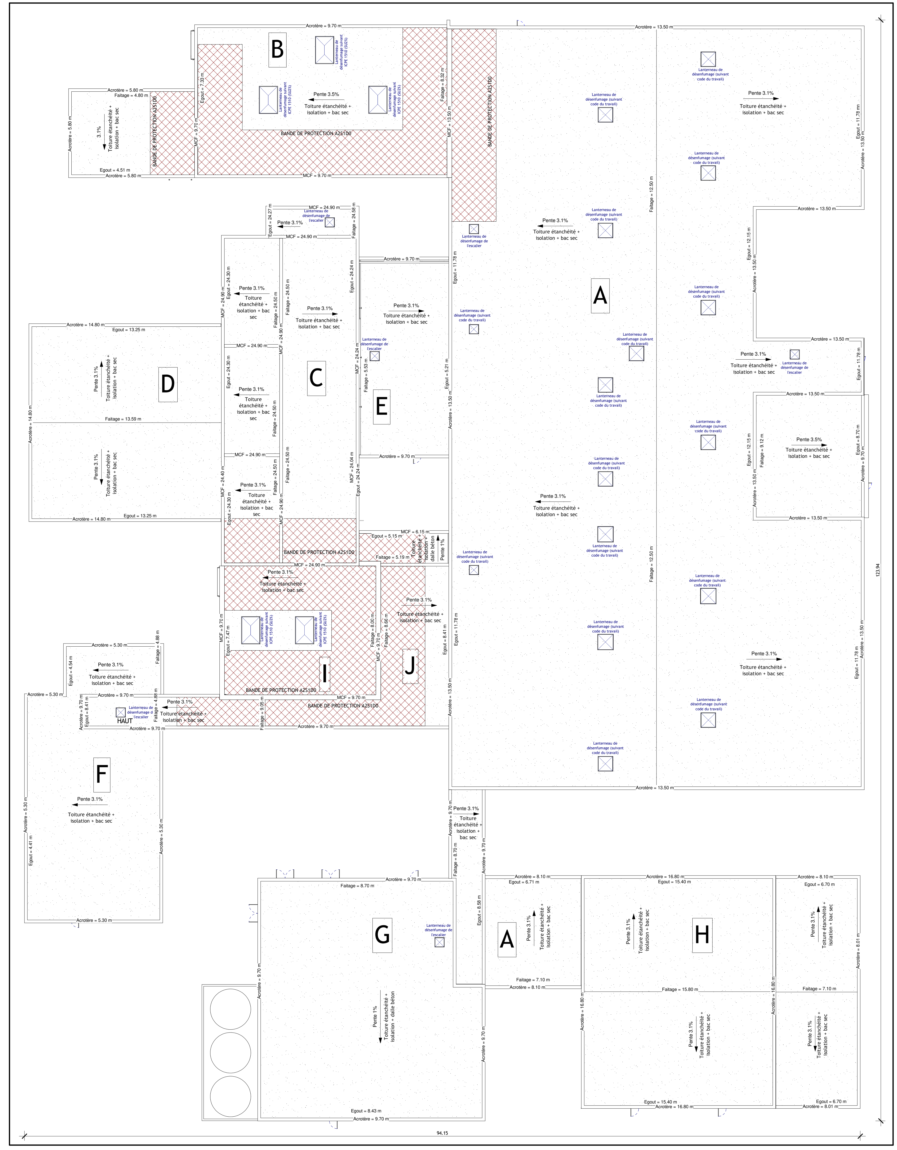
5 Plan de toitures Ech : 1 : 200
